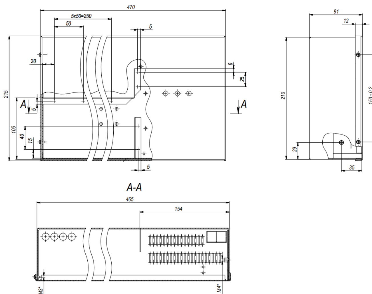
Рисунок 2 - Габаритный чертеж корпуса ТИП-3
